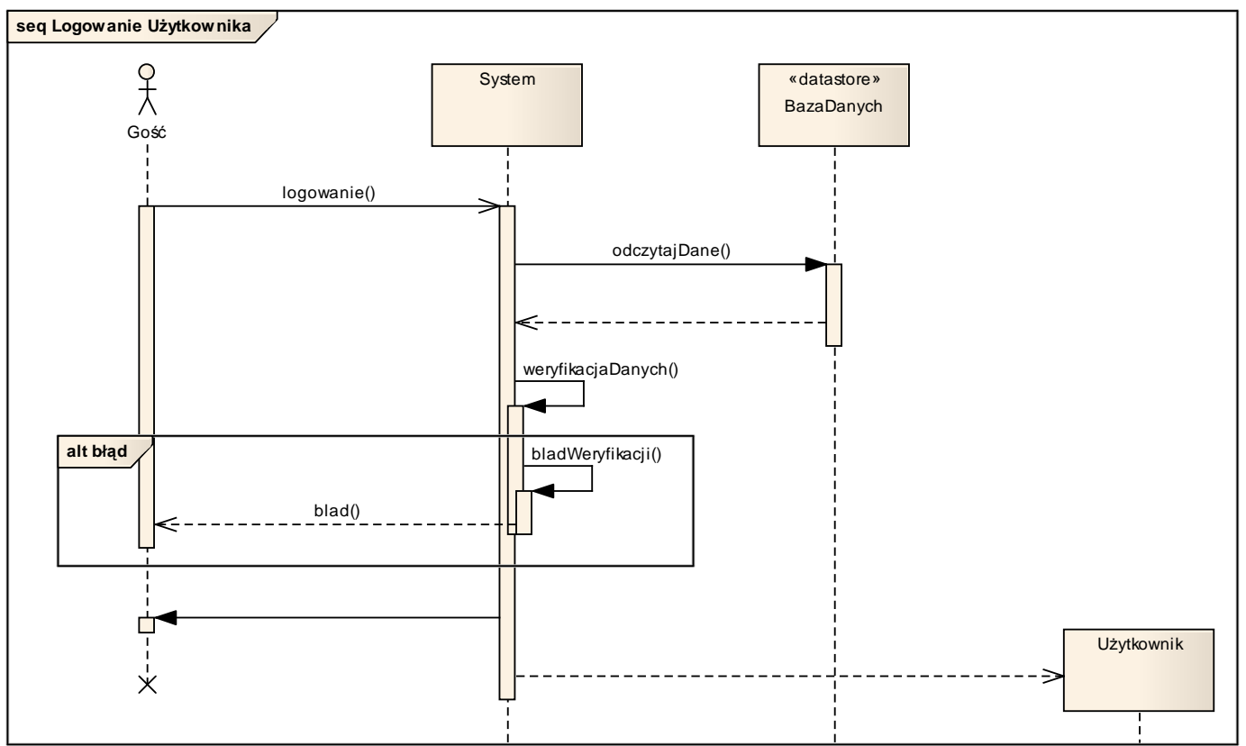
5.2 Diagram sekwencji - Logowanie użytkownika
