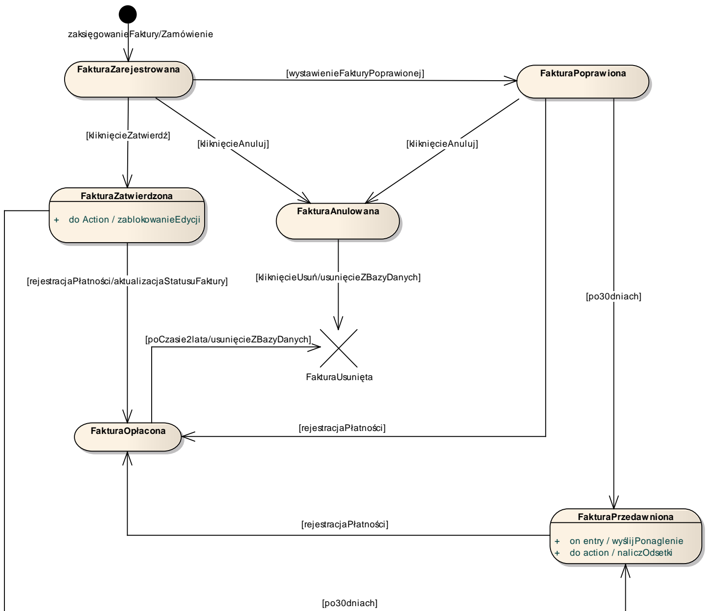
11.2 Diagram maszyny stanowej dla klasy Faktura
