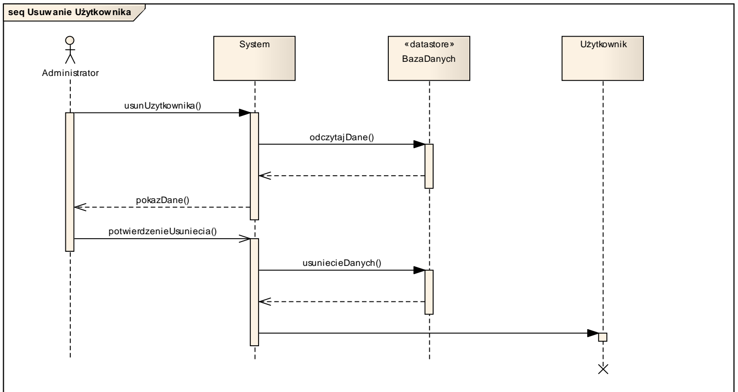
5.4 Diagram sekwencji - Usuwanie użytkownika
